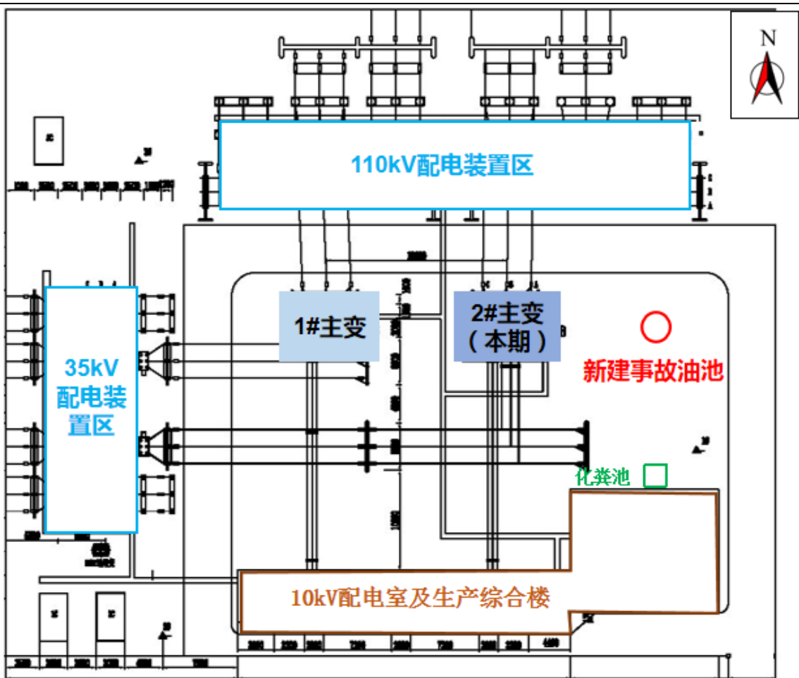
图 1-2 江永 110kV 变电站总平面布置图
