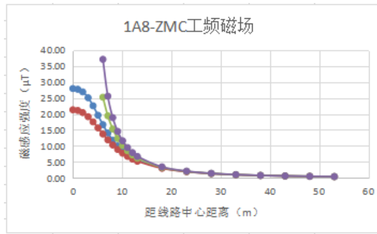
图3 110kV 单回线路（典型杆塔）磁感应强度预测分布图
