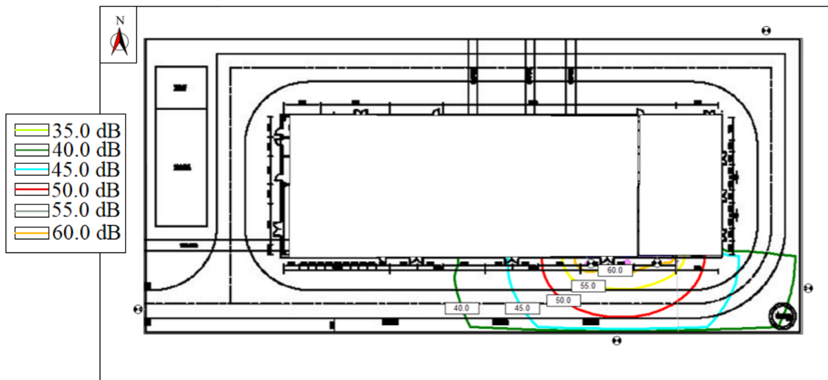
图 7-1 城西 110kV 变电站本期规模噪声预测等值线图
