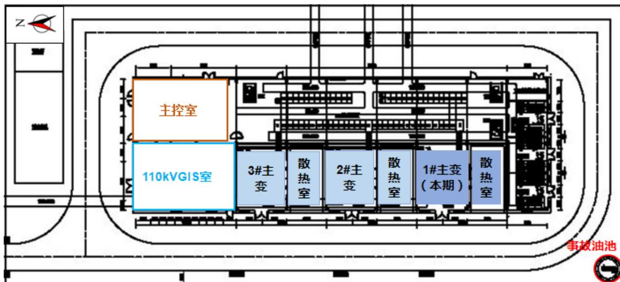
图 1-2 城西 110kV 变电站总平面布置示意
